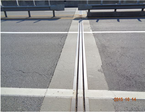
신축이음 전경
